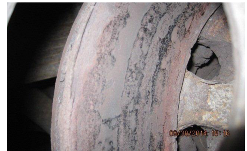
Disco Oxidado. Criterios de Fuera de Servicio, Parte II, a.(6)(d) o a.(7)(e) / 393.48(a)-EUA
