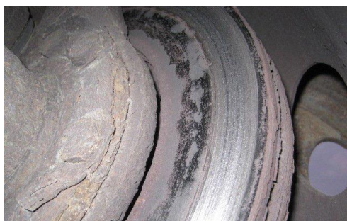
Contacto metal con metal. Criterios de Fuera de Servicio, Parte II, a.(6)(c) o a.(7)(d) / 393.48(a)-EUA.
